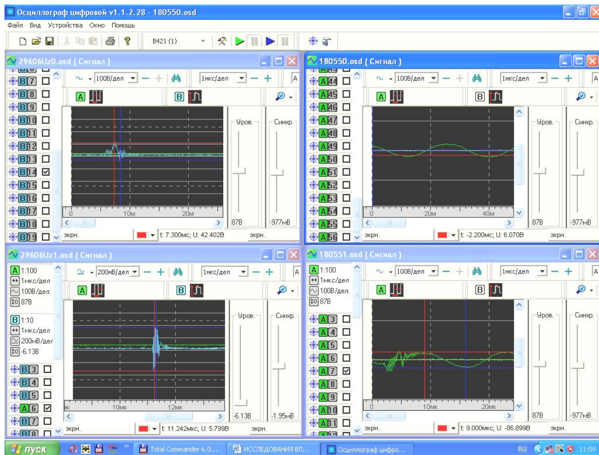
Рисунок 2 - Осциллограмма сигнала при пропускании УЗ через электролит при работе установки АМДО
