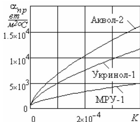
Рис. 1. Графики зависимости приведенного коэффициента теплоотдачи \alpha_{пр} от концентрации жидкости K для различных СОТС
