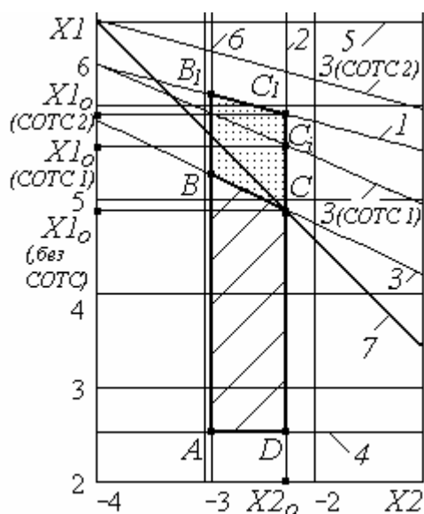
Рис 3. Схема определения оптимальных режимов резания для тонкого точения
